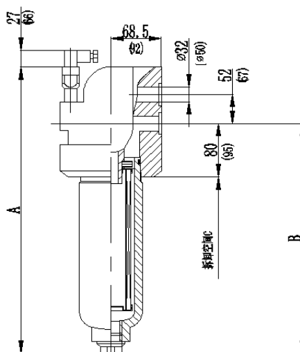
HP150-800连接尺寸及技术参数
