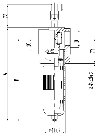
HL150-400连接尺寸及技术参数
