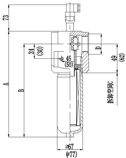
HL15-90连接尺寸及技术参数
