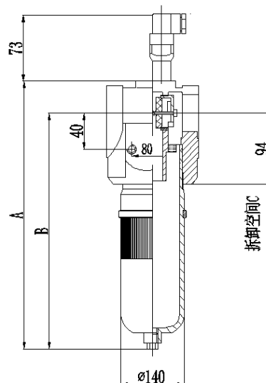
HL550-800连接尺寸及技术参数
